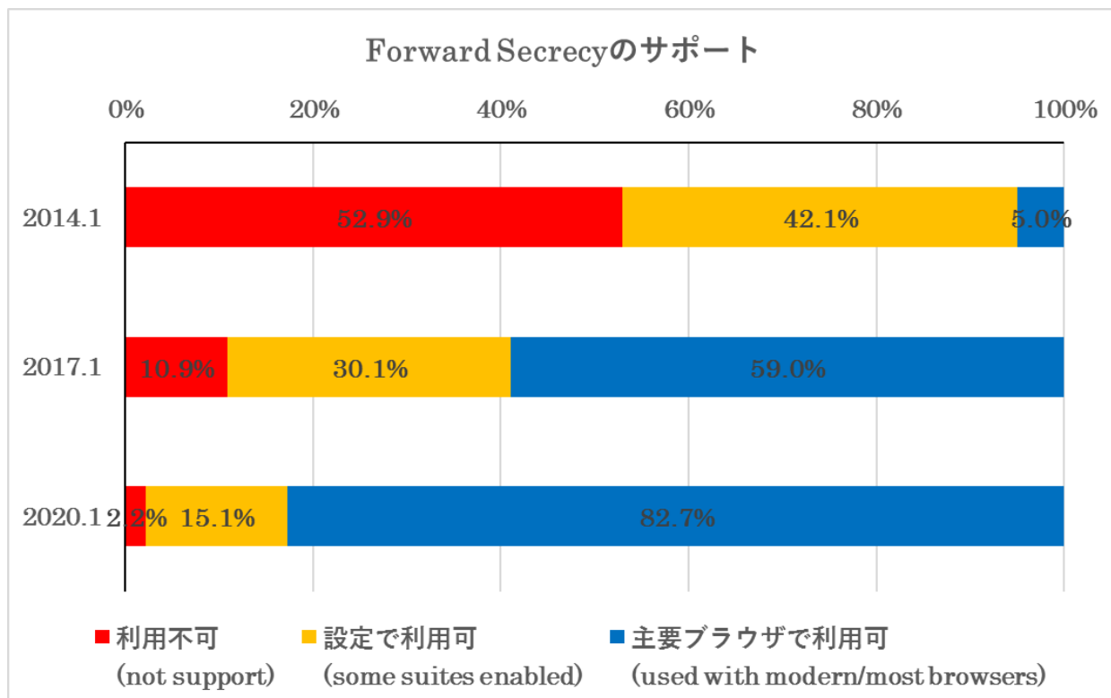
図 9 Perfect Forward Secrecy のサポート状況 (SSL Pulse による集計データを加工)
