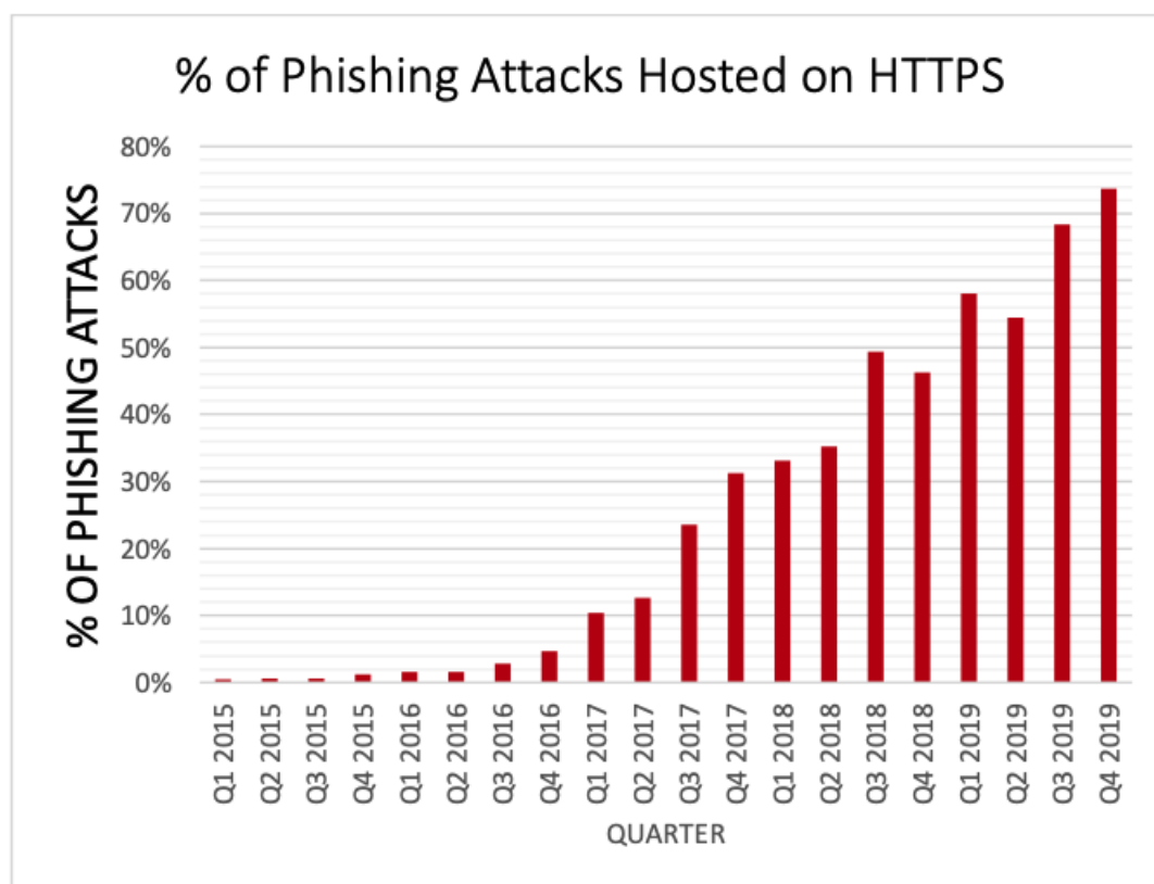
図 14 フィッシングサイトの HTTPS 利用率（[出典] The PhishLabs Blog [37] ）
