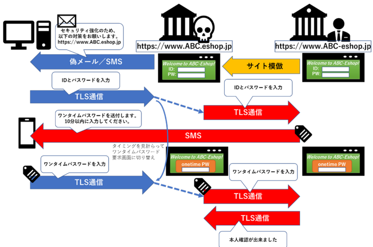
図 15 2 段階認証を突破するフィッシングの手手法例
