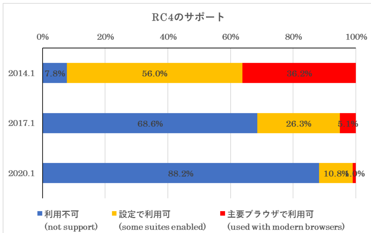
図 8 RC4 のサポート状況 (SSL Pulse による集計データを加工)
