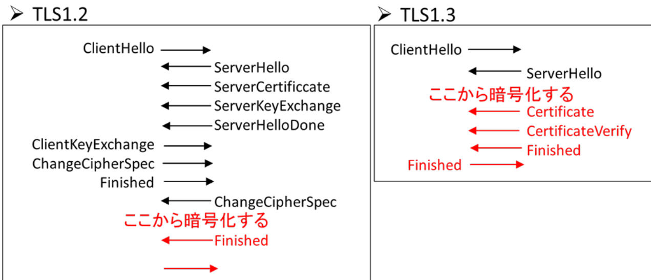
図 2 TLS1.2 と TLS1.3 との暗号化開始個所の比較
