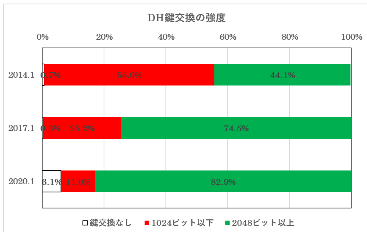
図 10 DH(E)鍵交換の鍵長の推移 (SSL Pulse による集計データを加工)
