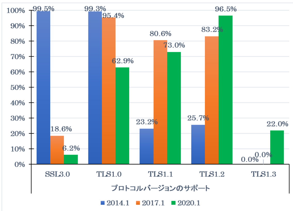
図 7 サポートされるプロトコルバージョンの推移 (SSL Pulse による集計データを加工)
